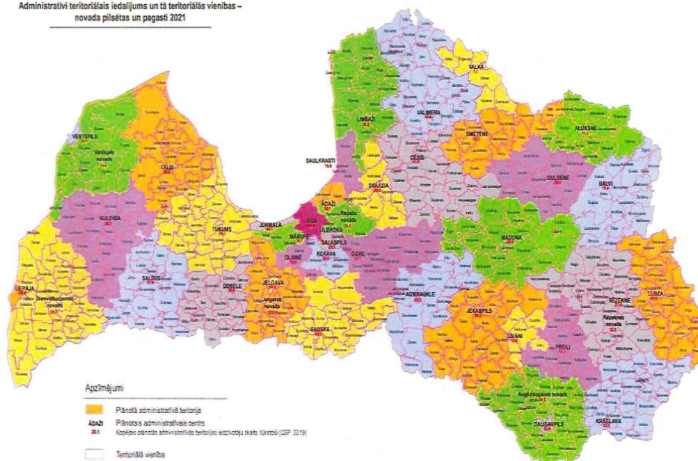
Administratīvi teritoriālais iedalījums un tā teritoriālās vienības – novada pilsētas un pagasti 2021
